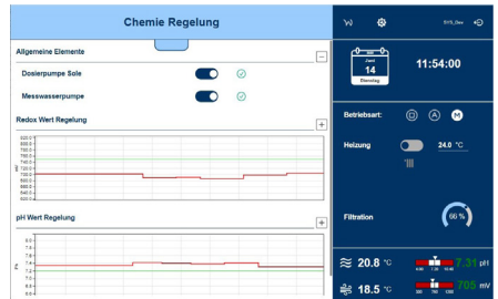
Abbildung: Übersicht Chemieregelung
