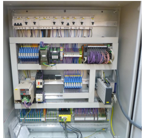
Abbildung: Schaltschrank - made in Switzerland
